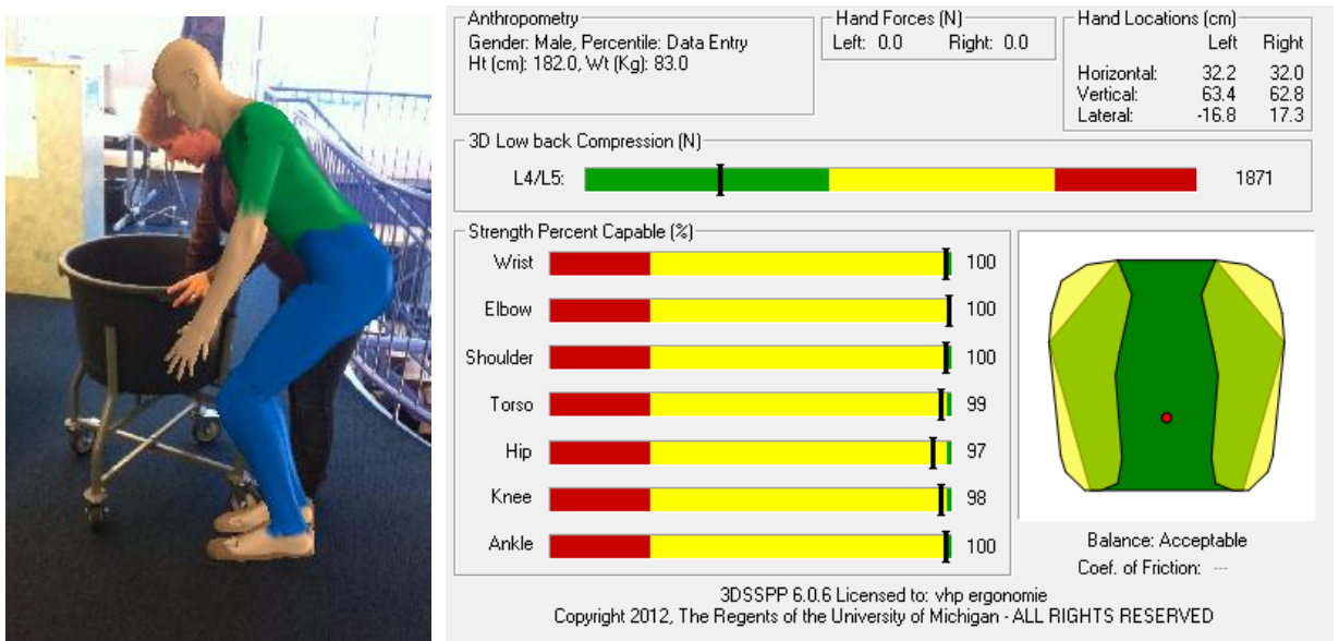
Figuur 2. 3DSSPP-model waarbij met de kuiphouder wordt gewerkt, 1871 N rugbelasting zonder tillen.
