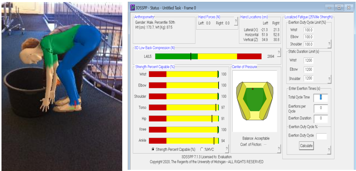
Figuur 1. 3DSSPP-model waarbij traditioneel wordt gewerkt, 2894 N rugbelasting zonder tillen.
